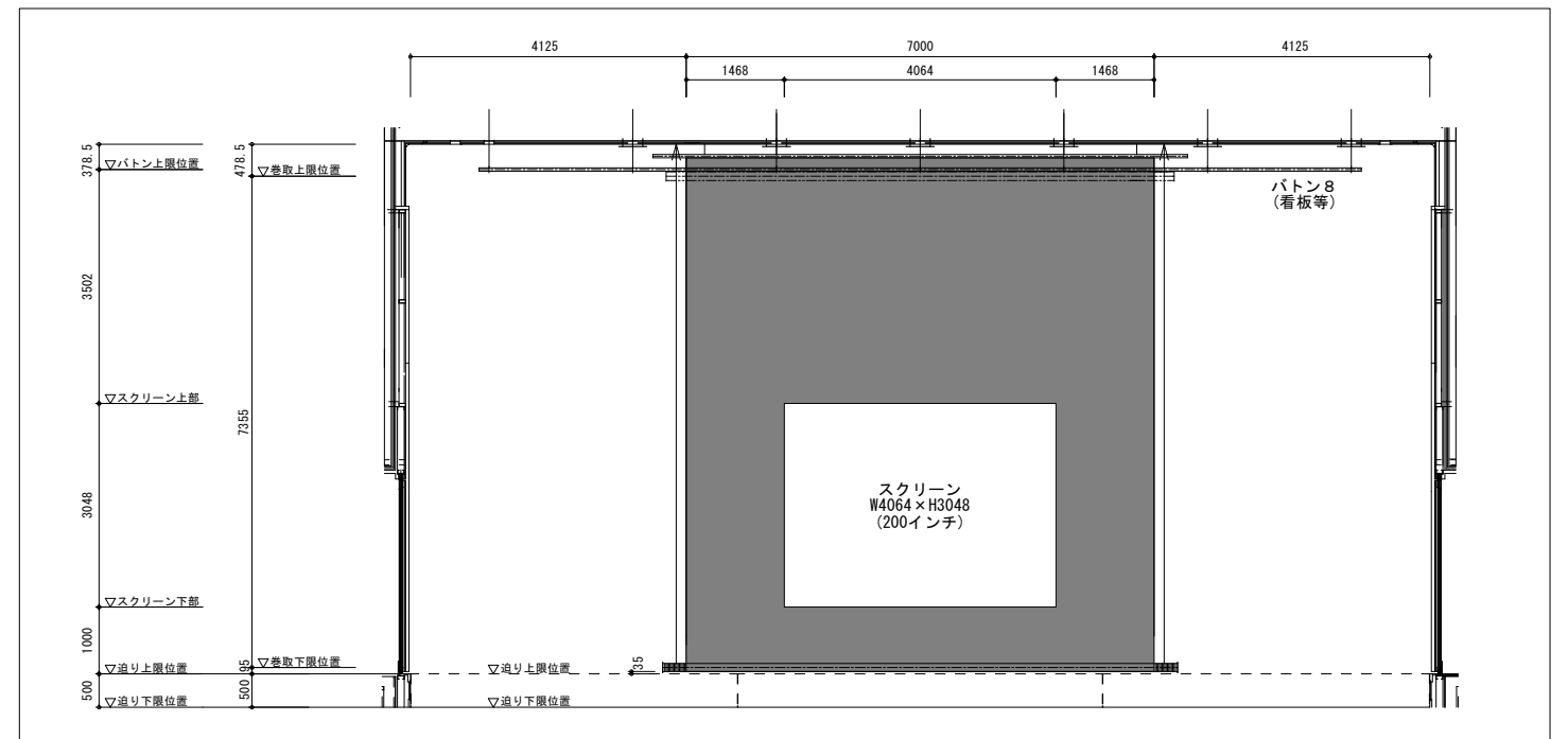
正面図
