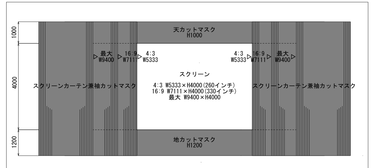
正面図
