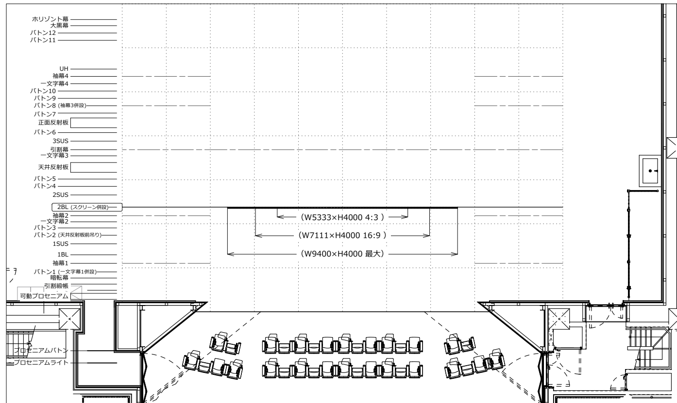
平面図
